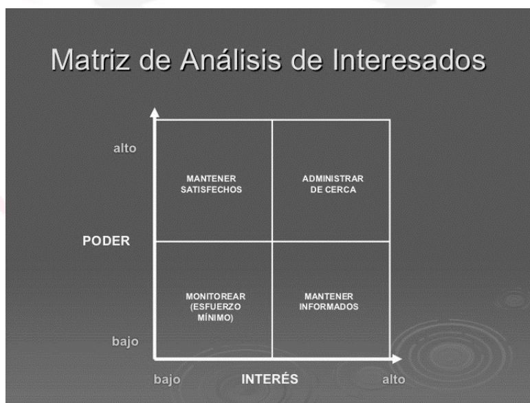
Ilustración 5.- Matriz de Interesados agrupados en niveles de poder e interés.
