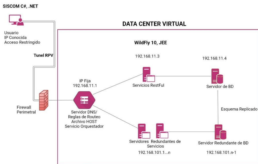
Ilustración 4.-Esquema SOA y Cliente Servidor propuesto.
